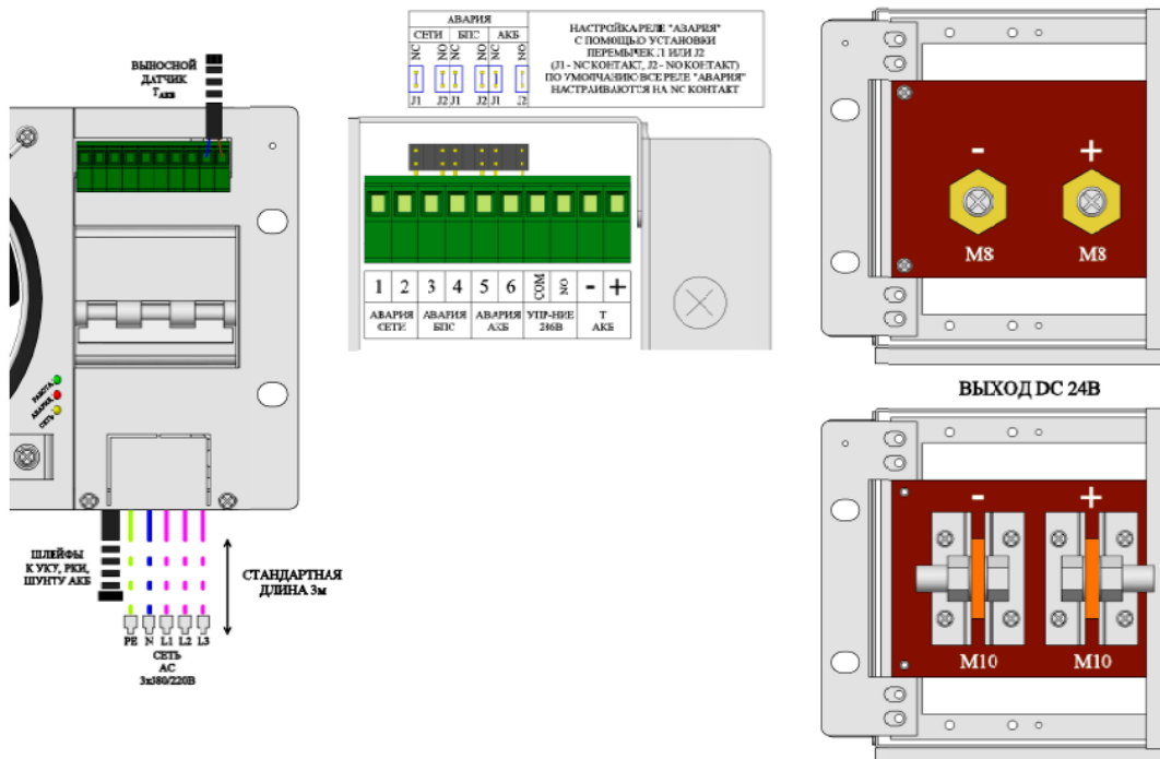
Рисунок 4. Распиновка силовых и сигнальных кабелей корзины ИПС-9000-380/24В-300А-0/3-3U.
