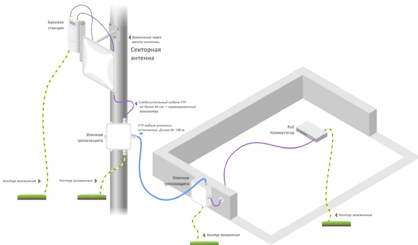
Рисунок 5 – Схема подключения базовой станции для обеспечения грозозащиты
