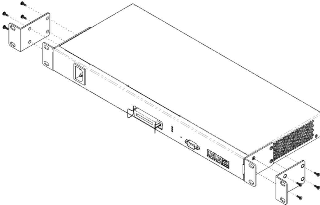
Рисунок 6 – Крепление кронштейнов
