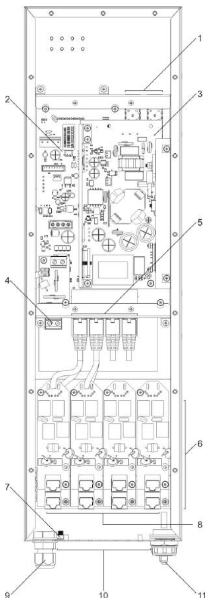
Рисунок 42 – Основные компоненты и разъемы MES3708P
