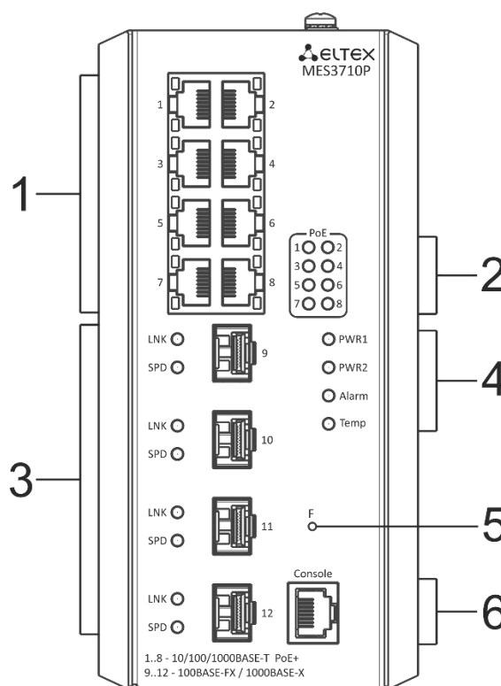
Рисунок 28 – Передняя панель MES3710P
