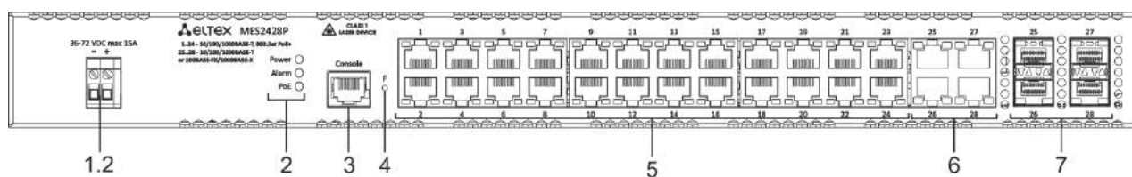
Рисунок 15 – Передняя панель MES2428P DC
