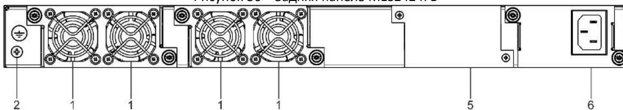
Рисунок 37 — Задняя панель MES3400-24, MES3400-48
