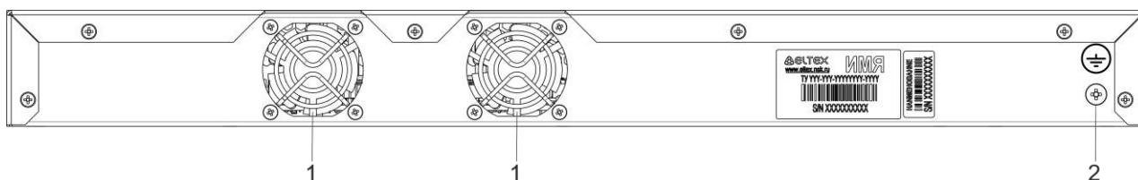
Рисунок 35 – Задняя панель MES2411X
