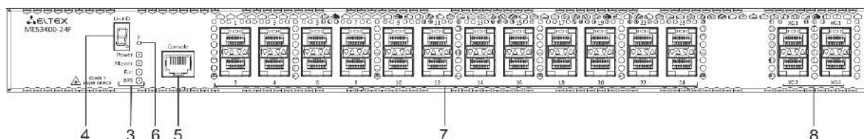
Рисунок 27 — Передняя панель MES3400-24F
