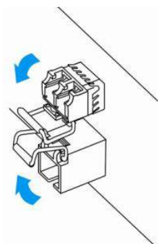
Рисунок 53 – Открытие защелки SFP-трансиверов
