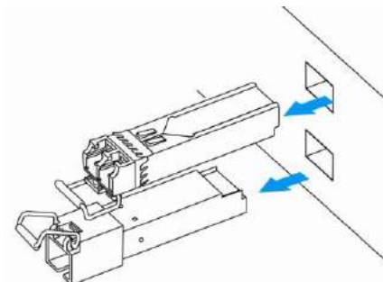
Рисунок 54 – Извлечение SFP-трансиверов
