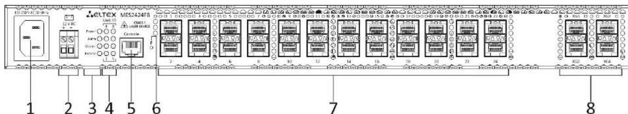
Рисунок 26 — Передняя панель MES2424FB
