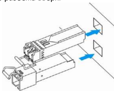
Рисунок 51 – Установка SFP-трансиверов
