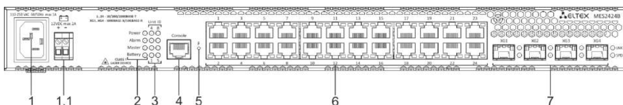
Рисунок 18 – Передняя панель MES2424B
