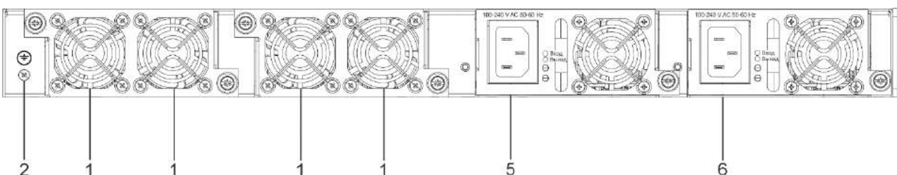
Рисунок 34 – Задняя панель MES2448P
