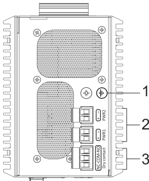
Рисунок 39 — Верхняя панель MES3710P
