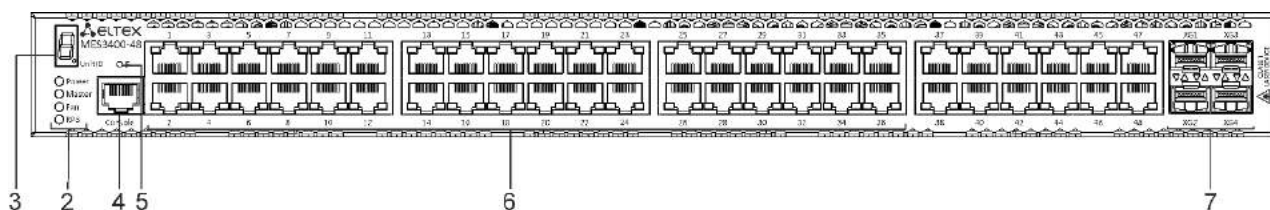
Рисунок 25 – Передняя панель MES3400-48
