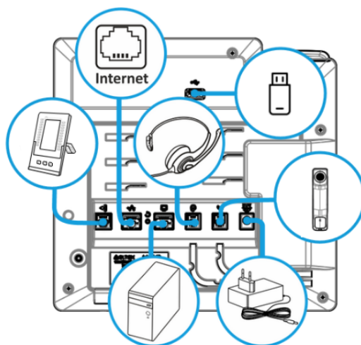
Схема включения VP-20(P)
