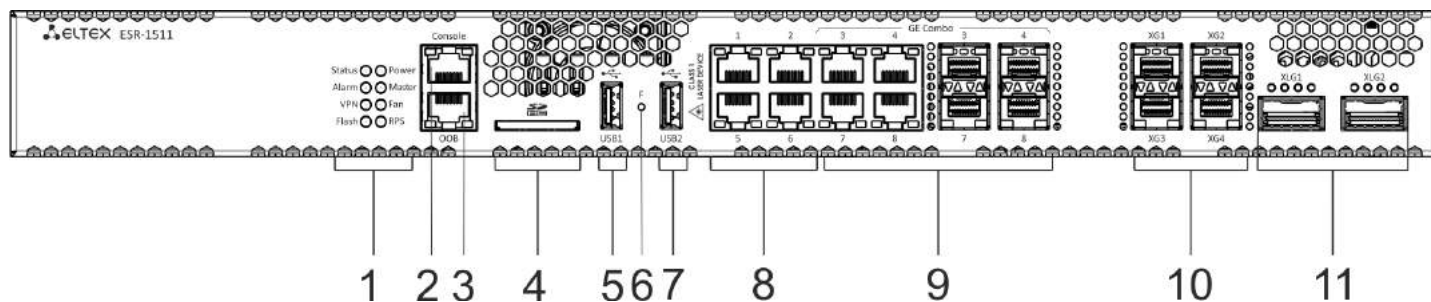
Рисунок 17 – Передняя панель ESR-1511
