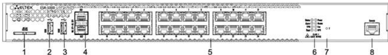
Рисунок 23 – Передняя панель ESR-1000
