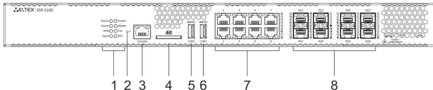
Рисунок 9 – Передняя панель ESR-3100
