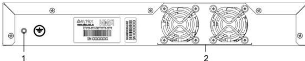
Рисунок 29 – Задняя панель ESR-200, ESR-100
