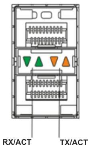
Рисунок 55 – Расположение индикаторов оптических интерфейсов
