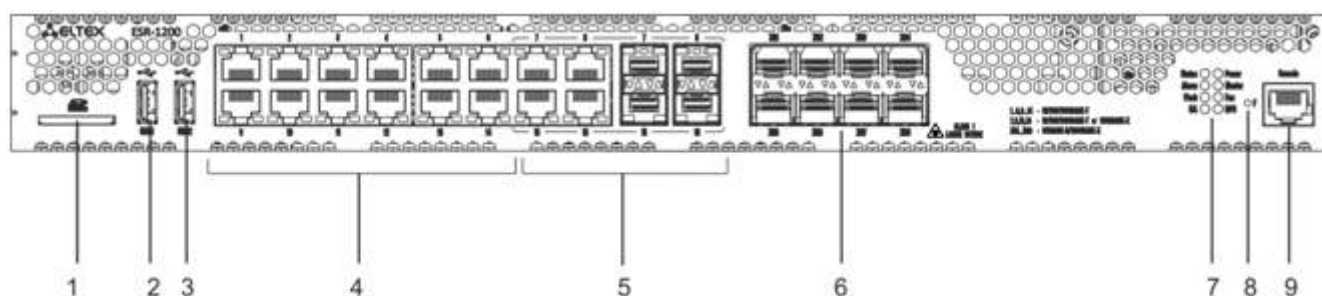
Рисунок 22 – Передняя панель ESR-1200
