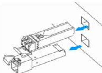
Рисунок 72 – Извлечение SFP-трансиверов
