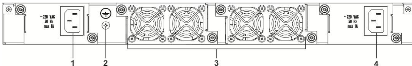
Рисунок 19 – Задняя панель ESR-1511, ESR-1500
