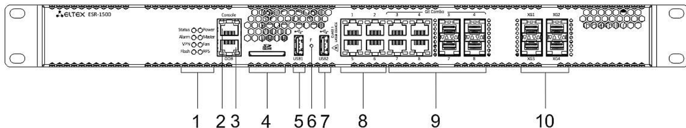
Рисунок 18 – Передняя панель ESR-1500
