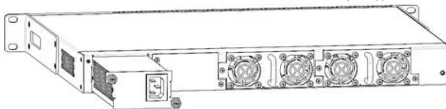
Рисунок 67 – Установка модулей питания
