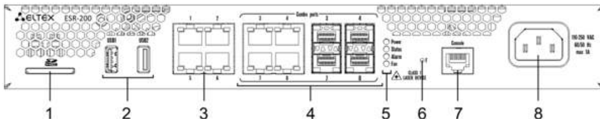
Рисунок 27 – Передняя панель ESR-200
