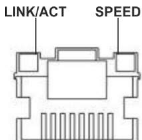
Рисунок 54 – Расположение индикаторов разъема RJ-45
