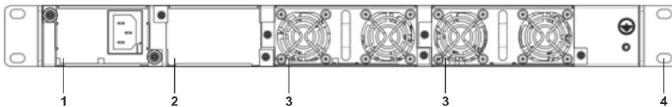
Рисунок 24 – Задняя панель ESR-1000
