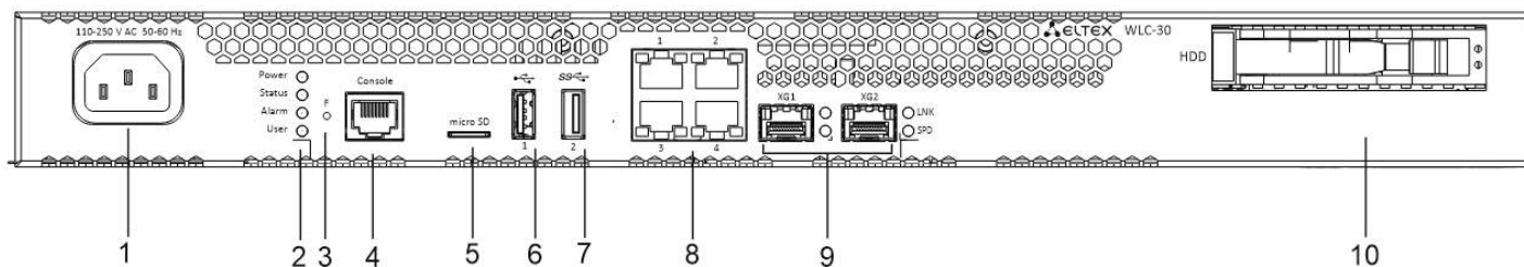
Рисунок 1 – Передняя панель WLC-30
