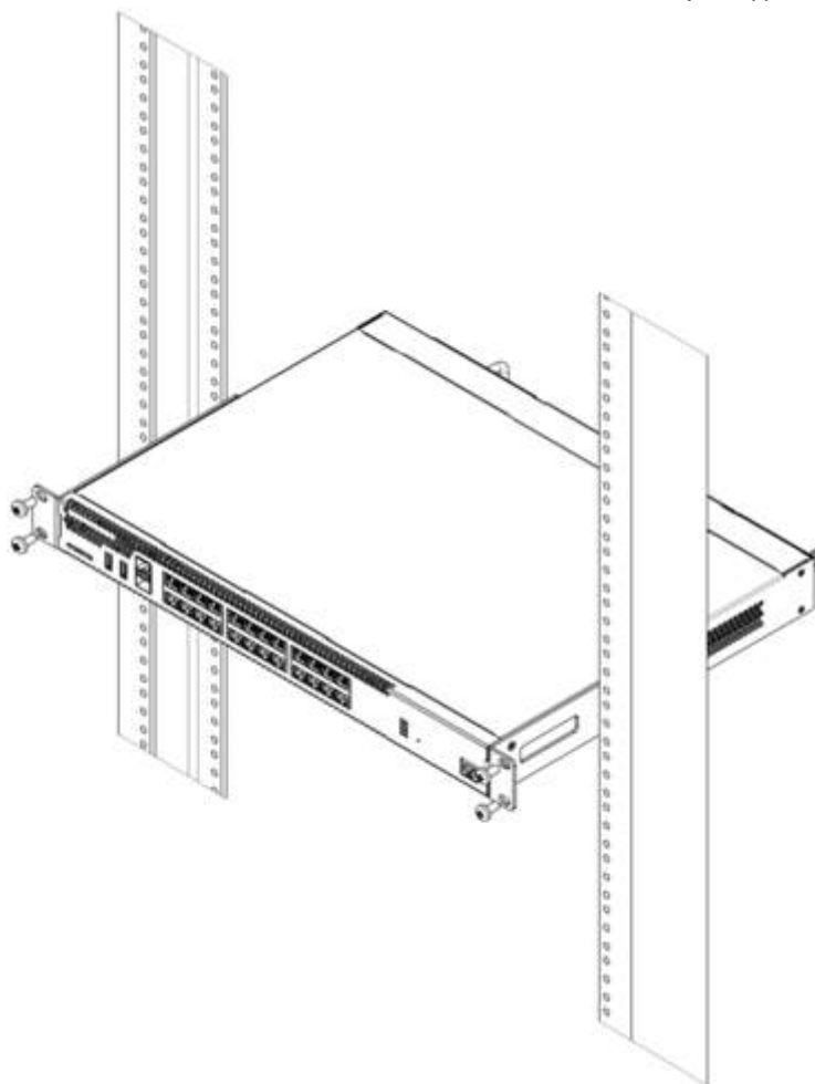
Рисунок 66 – Установка устройства в стойку
