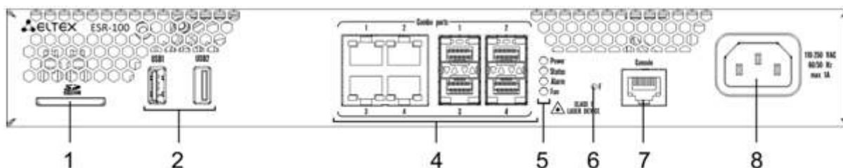
Рисунок 28 – Передняя панель ESR-100
