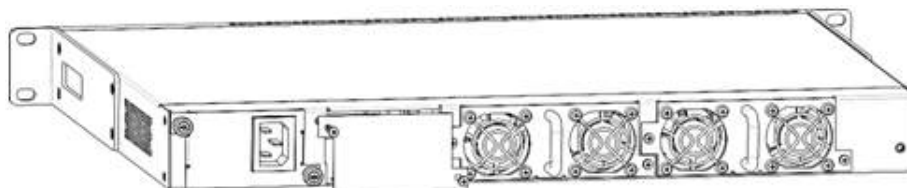
Рисунок 68 – Установка заглушки
