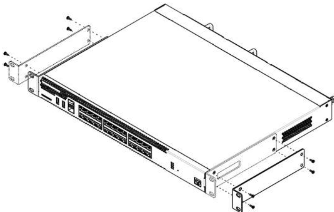
Рисунок 65 – Крепление кронштейнов
