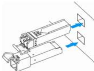
Рисунок 69 – Установка SFP-трансиверов
