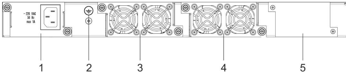
Рисунок 10 – Задняя панель ESR-3100
