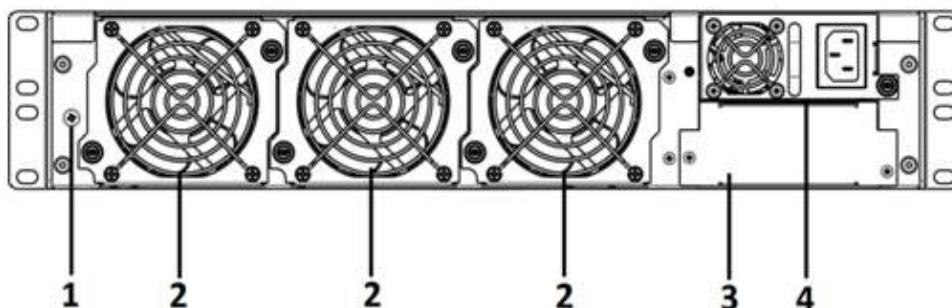
Рисунок 14 – Задняя панель ESR-1700
