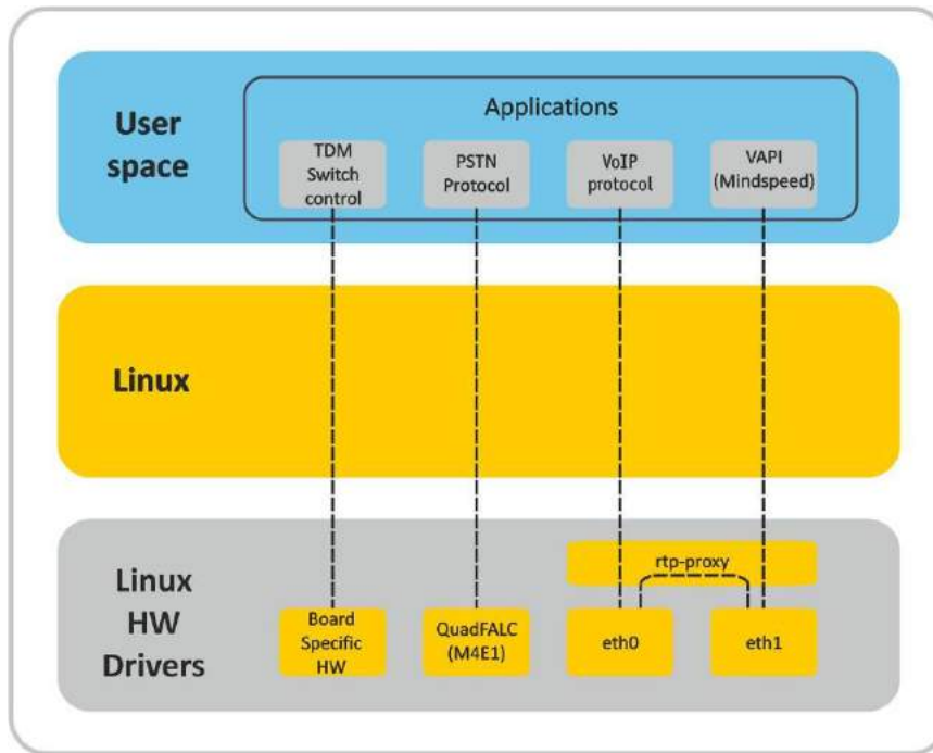
Рисунок 6 – Структура программного обеспечения SMG
