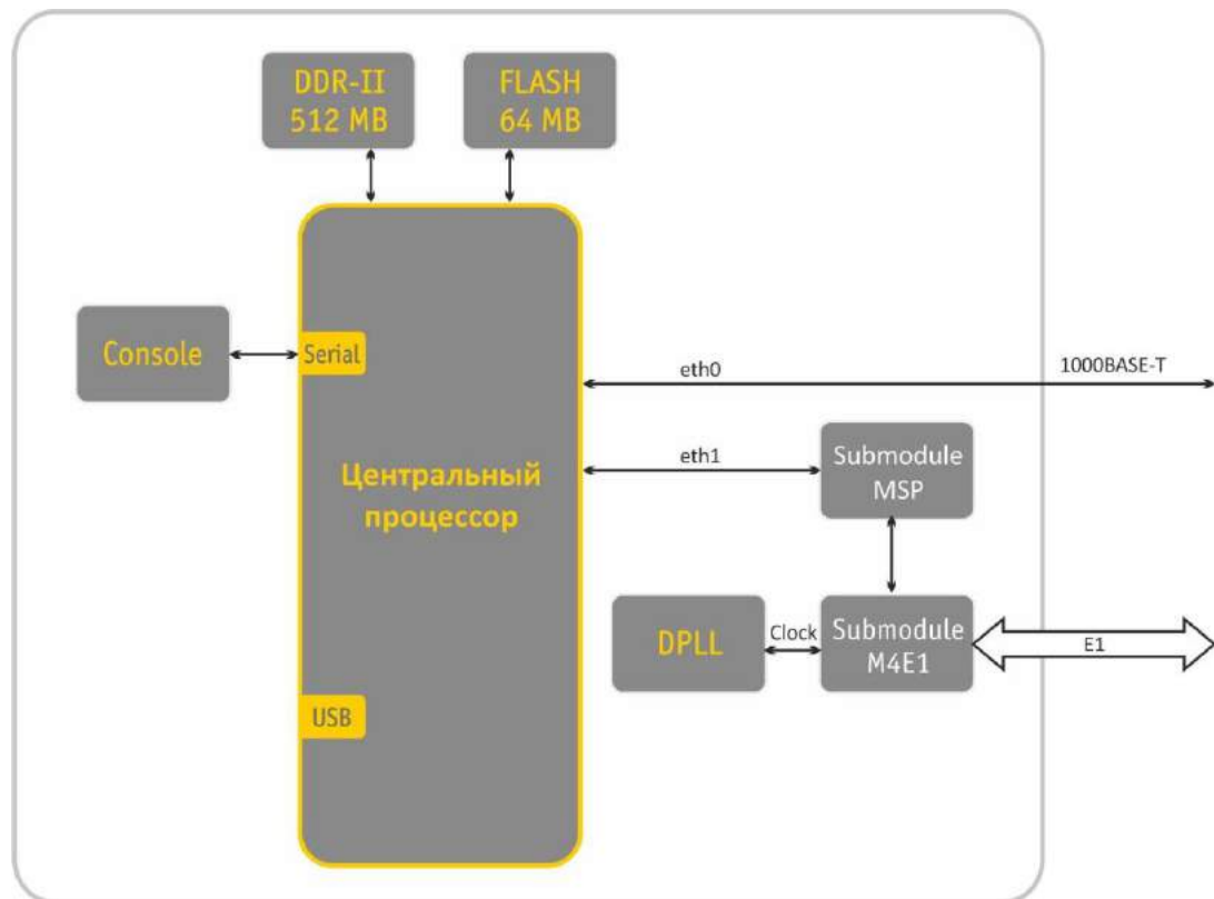
Рисунок 5 – Функциональная схема SMG
