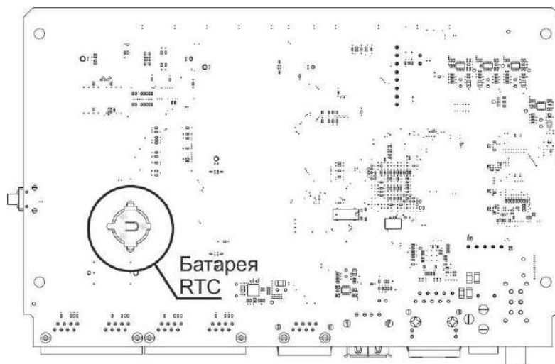
Рисунок 10 – Положение батареи RTC
