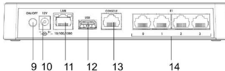
Рисунок 8а – Внешний вид SMG-4. Задняя панель
