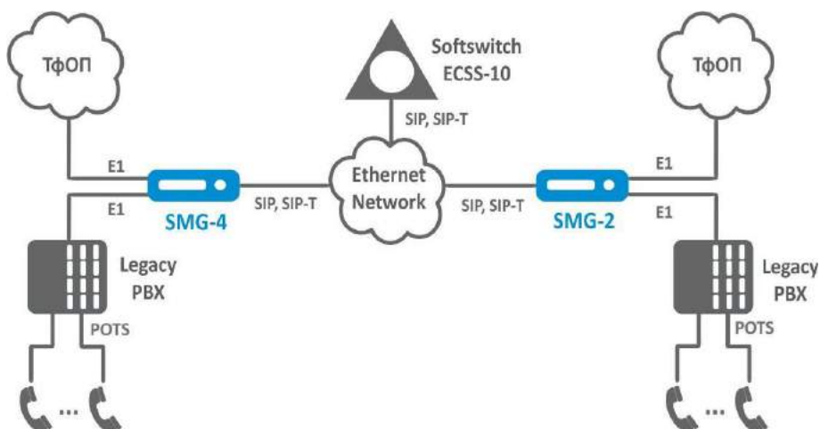
Рисунок 3 – Сопряжение сигнализации и медиапотоків TDM- и VoIP-сетей
