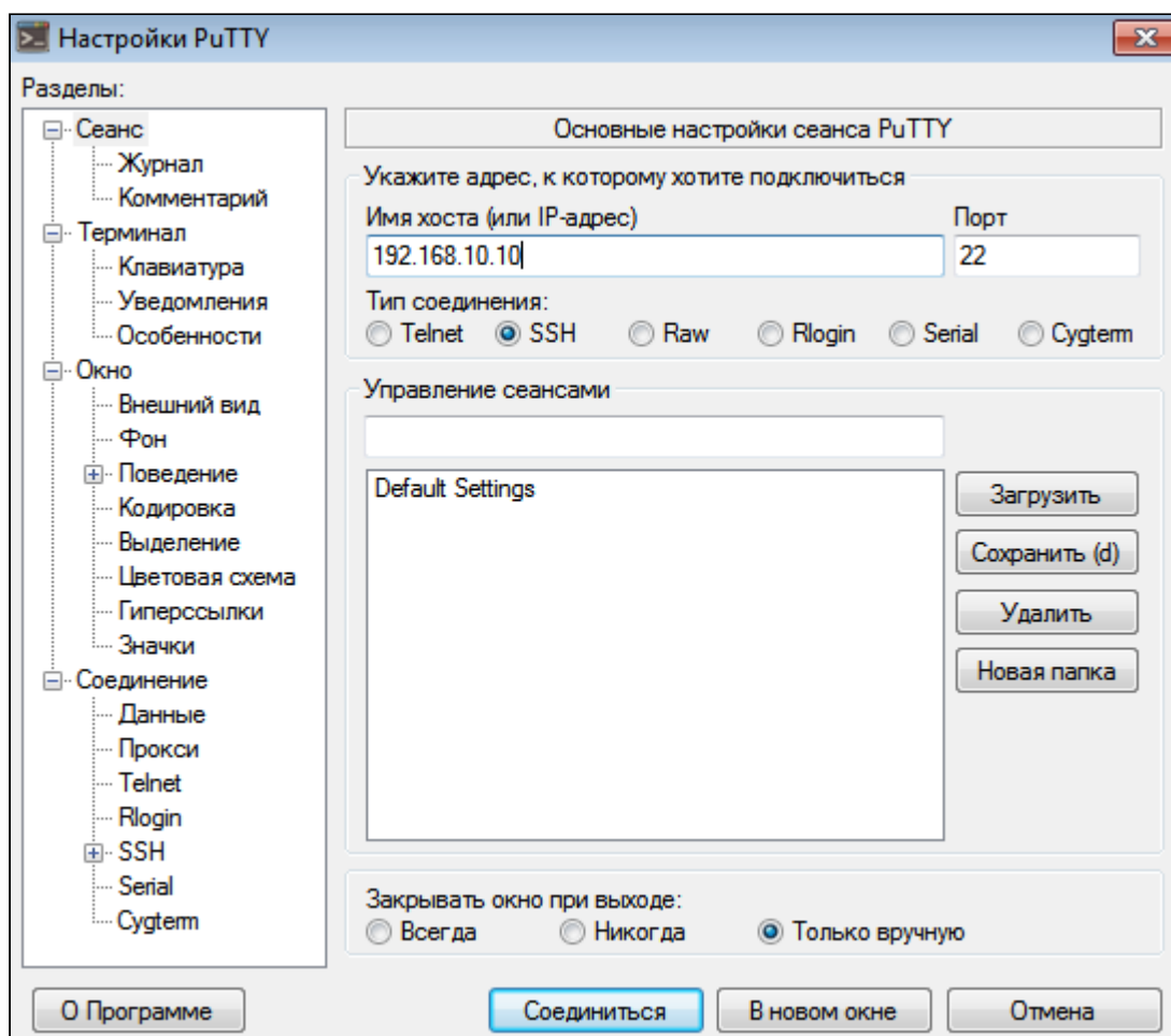
Рисунок 11 – Запуск SSH-клиента
