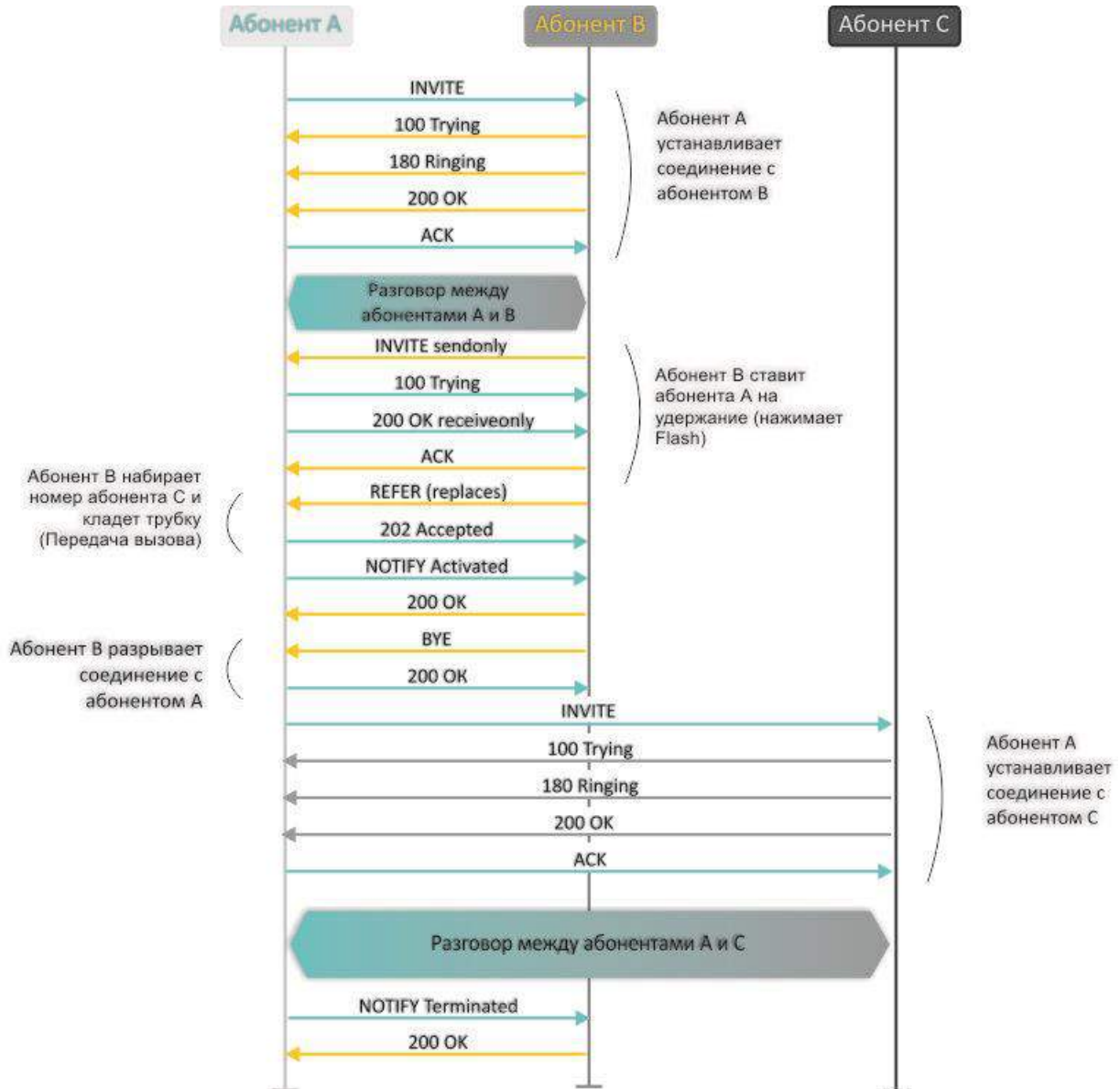
Рисунок 11 – Алгоритм выполнения услуги «Перевод вызова без сопровождения» («Unattended calltransfer») абонентом «В» по протоколу SIP
