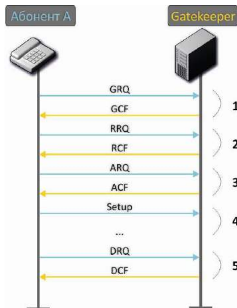
Рисунок 20 – Алгоритм вызова через гейткипер
