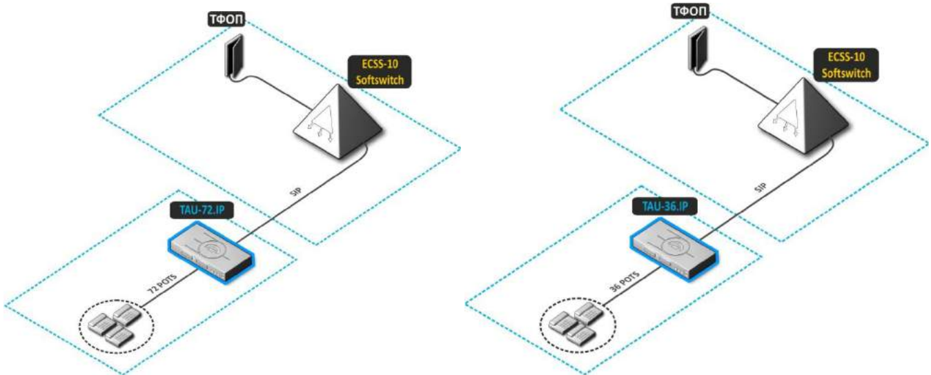
Рисунок 1 – Абонентский вынос TAU-72.IP/TAU-36.IP
